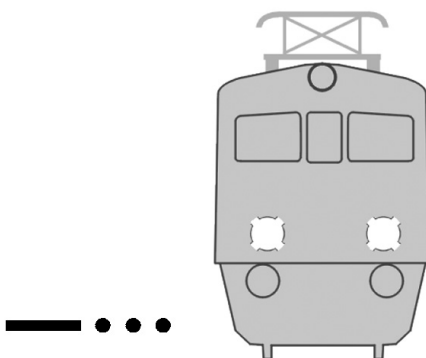
Rys. 147. Sygnał A 1
