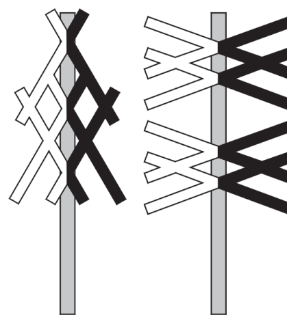
Rys. 195. Wskaźnik W 13
