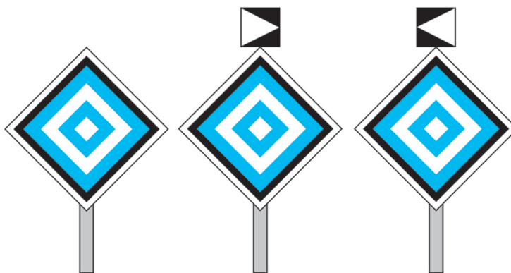
Rys. 202. Wskaźniki We 4a, We 4b, We 4c
