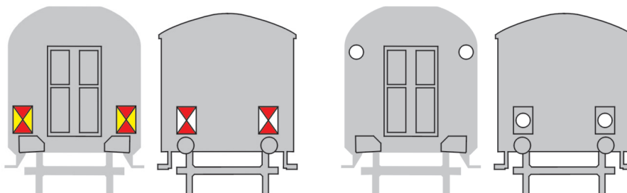
Rys. 135. Sygnał Pc 4 (dzienny), Pc 5 (dzienny)
