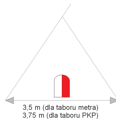
Rys. 43 Wskaźnik W 17
