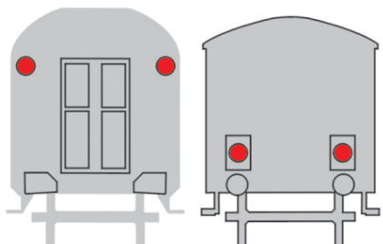
Rys. 137. Sygnał Pc 5 (dzienny i nocny)
