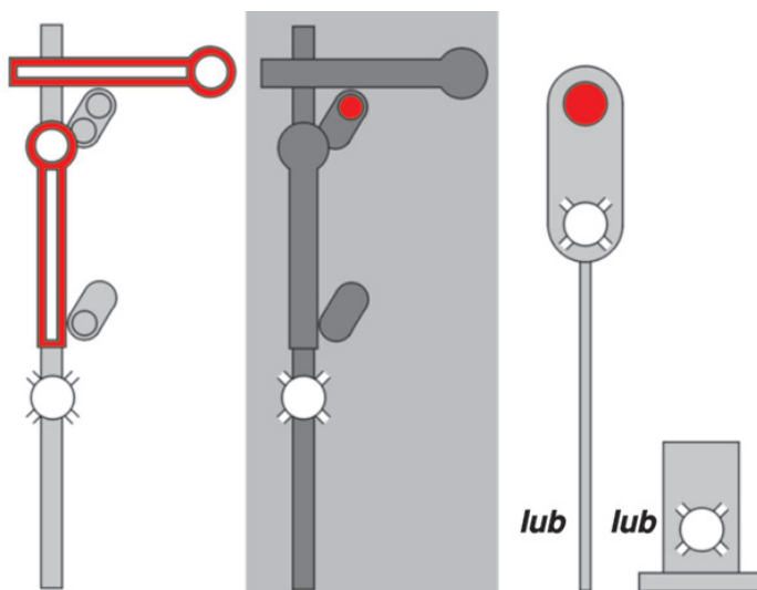
Rys. 24. Sygnał Sz
