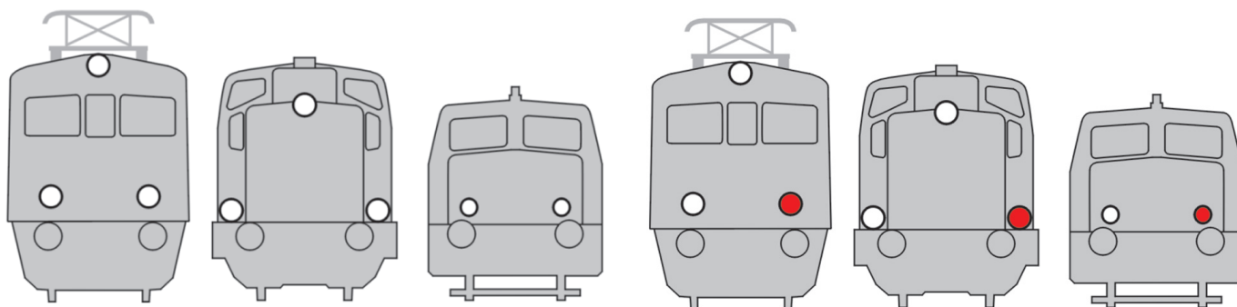
Rys. 132. Sygnał Pc 1 (dzienny i nocny)
