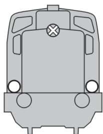
Rys. 134. Sygnał Pc 3 (dzienny i nocny)
