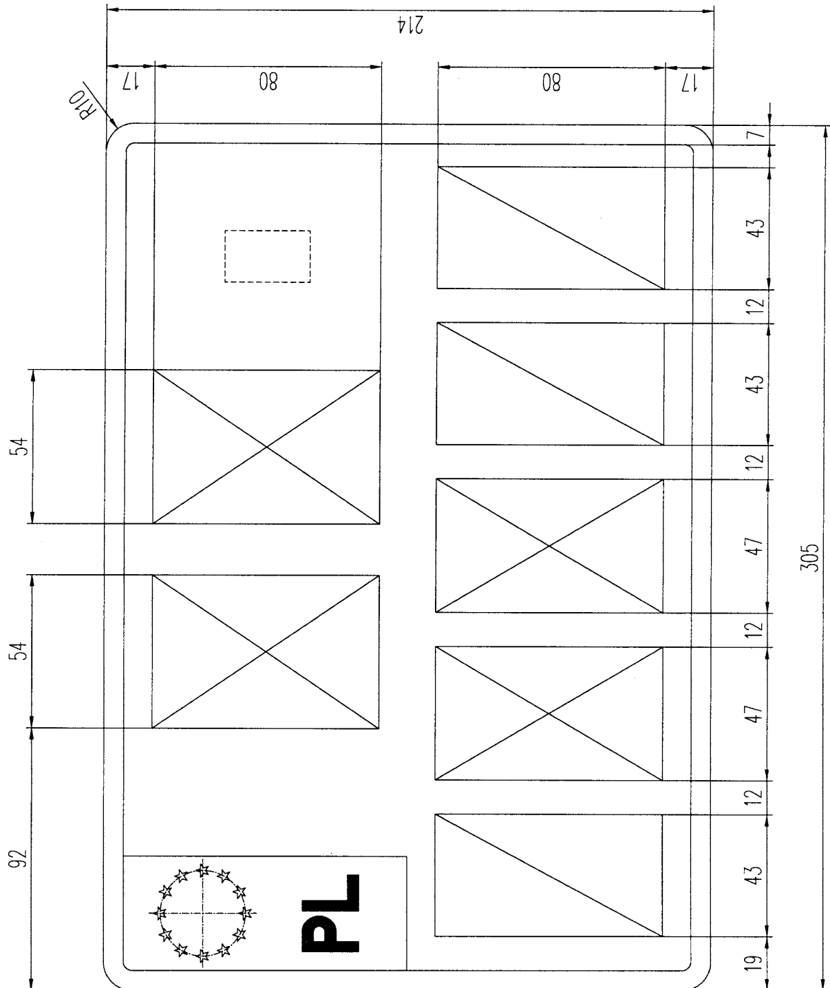
Rysunek 21b. Tablica samochodowa zwyczajna dwurzędowa (2 litery, 1 cyfra, 1 cyfra, 2 litery, 2 cyfry)
