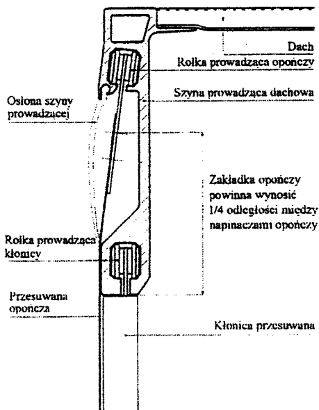
Rysunek nr 9.2 Prowadnica oponczy i zakładka górna oponczy
