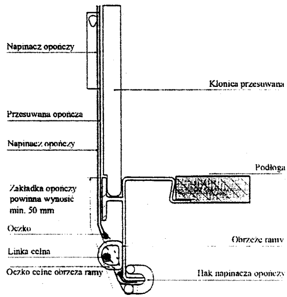
Rysunek nr 9.3 Zakładka dolna oponczy
