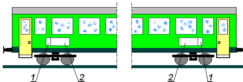
Rys. 6. Wzór rozmieszczenia tablic kierunkowych i numerowych zewnętrznych na wagonie kursującym w przewozach międzywojewódzkich:
