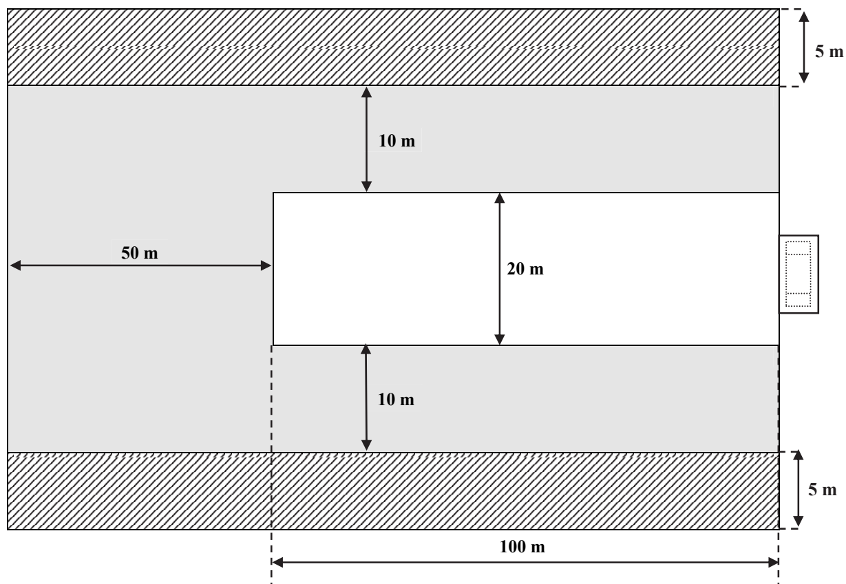
Rys. 1. Płyta poślizgowa w kształcie prostokąta wraz ze strefami bezpieczeństwa, stanowiąca element infrastruktury ośrodka doskonalenia techniki jazdy stopnia wyższego
