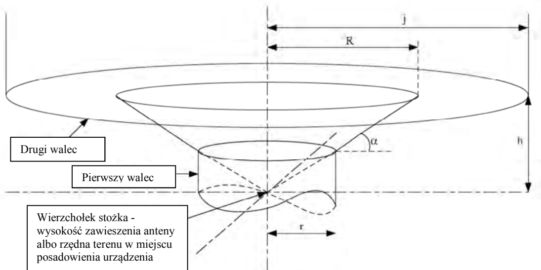
Rys. 1. Kształt powierzchni ograniczających zabudowę wokół dookólnych lotniczych urządzeń naziemnych – widok trójwymiarowy*
