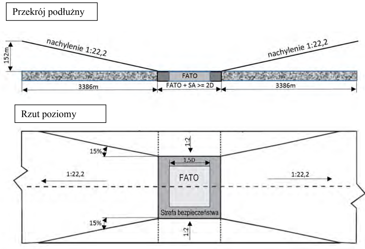
Rysunek 8. Schemat i zakres powierzchni ograniczających wysokość obiektów naturalnych i sztucznych w otoczeniu lądowiska wyniesionego dla śmigłowców z kierunków podejścia i wznoszenia
