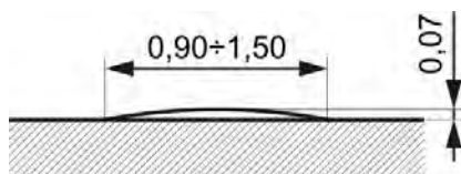
Rys. 8.1.5. Kształt i wymiary liniowego progów zwalniającego listwowego U-16d o ograniczonej prędkości przejazdu 18–20 km/h
