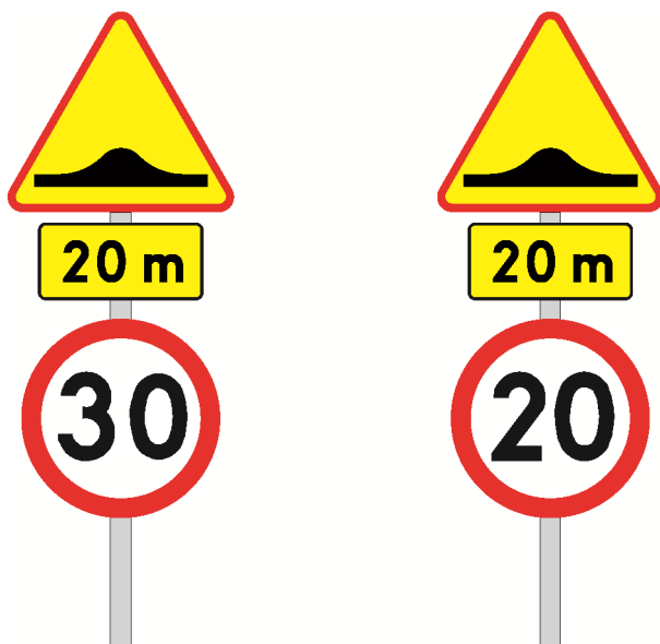
Rys. 8.1.10. Oznakowanie pionowe progów zwalniających:
