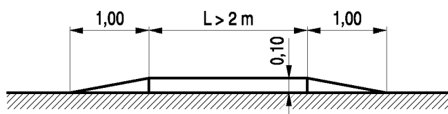
Rys. 8.1.3. Kształt i wymiary liniowego progów zwalniającego płytowego U-16c o ograniczonej prędkości przejazdu 25–30 km/h
