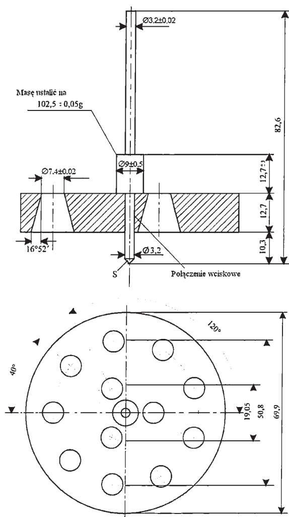
Rysunek 1 Penetrometr
