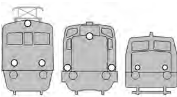
Rys. 132. Sygnał Pc 1 (dzienny i nocny)
