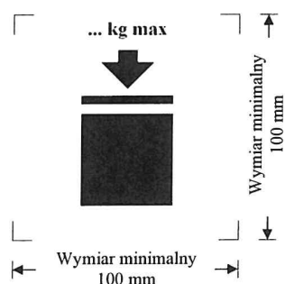
Rys. 6.5.2.2.2.1
