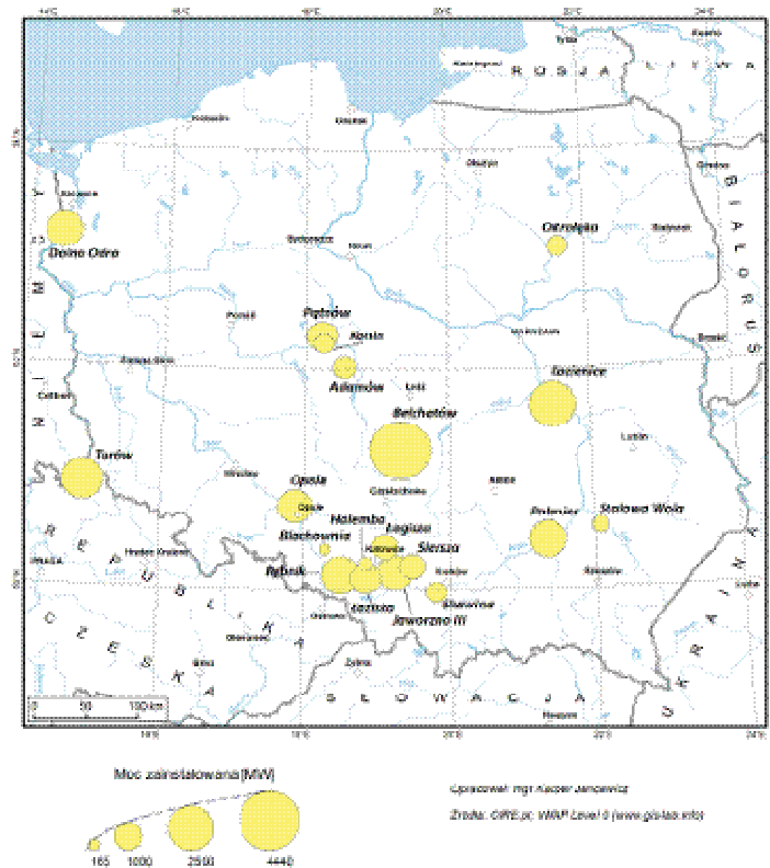
Rysunek 3. Istniejące w 2012 r. elektrownie ciepłowne w Polsce
