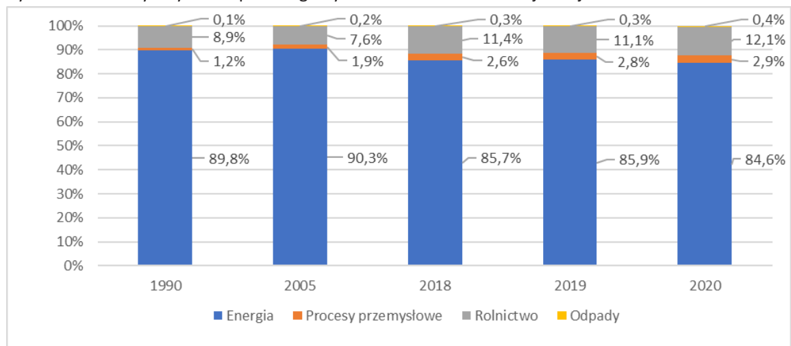
Rysunek 6. Historyczny udział poszczególnych sektorów w całkowitej emisji NO x
