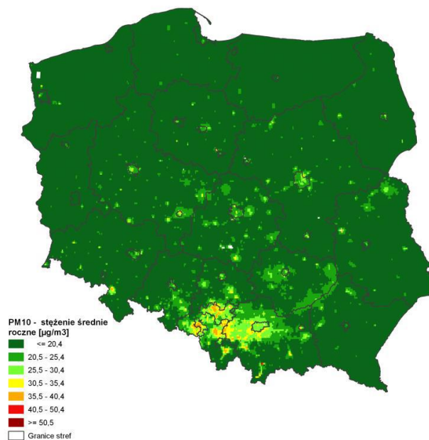
Rysunek 19. Rozkład przestrzenny średniego rocznego stężenia PM10 na obszarze Polski w 2020 r., określony na podstawie modelowania matematycznego oraz obiektywnego szacowania
