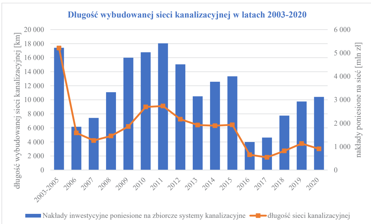
Wykres 3. Długość wybudowanej sieci kanalizacyjnej w latach 2003-2020
