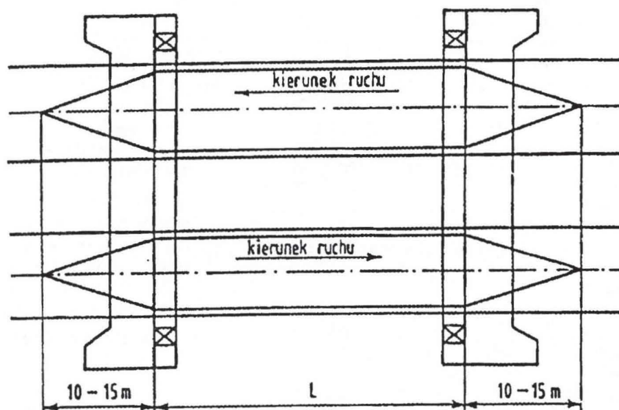
Rys. 3.3 Schemat układania odbojnic na obiektach inżynieryjnych
