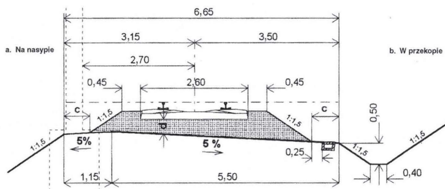
Rys. 3.2 c Przekrój normalny toru — linia magistralna i pierwszorzędna jednotorowa na prostej
