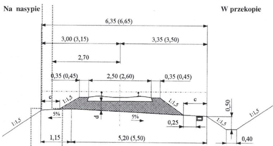
Rys. 3.2 e Przekrój normalny toru — linia drugorzędna i znaczenia miejscowej jednotorowa na prostej
