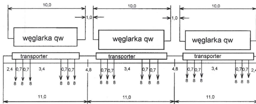
Rys. 4.3 Schematy obciążeń obiektów inżynieryjnych
