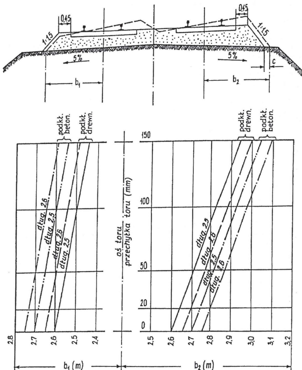
Rys. 3.2 f Wyznaczanie dolnej krawędzi podsypki w torze z przechylką na linii dwutorowej przy zasypaniu czół podkładów na szerokości 0,45 m, z zastrzeżeniem, że:
