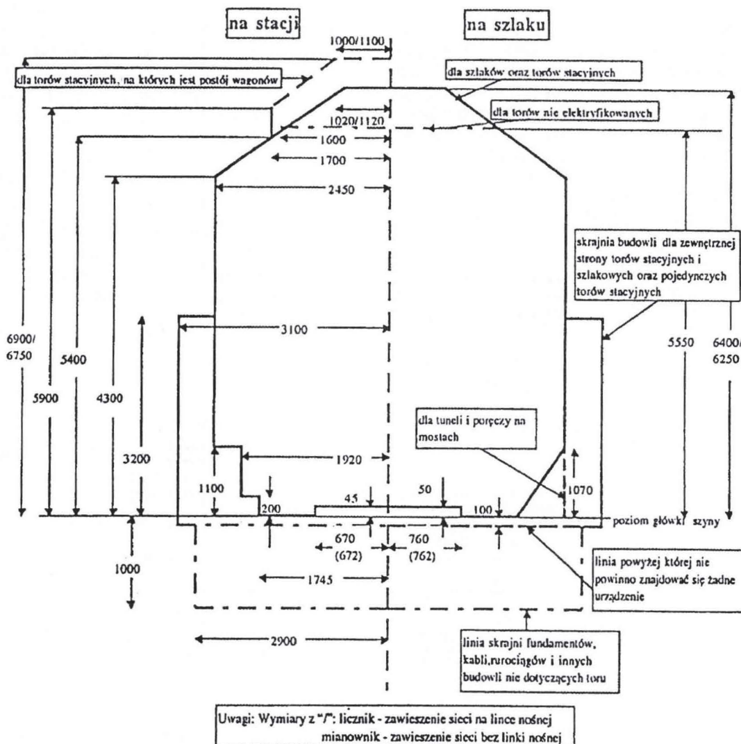
Rys. 5.1 Skrajnia budowli dla torów szerokich 1520 (1524) mm według normy GOST 9238 — 83 /Gosudarstwiennyj Standart Sojuza SSR/
