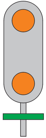
Rys. 15. Sygnał S 9
