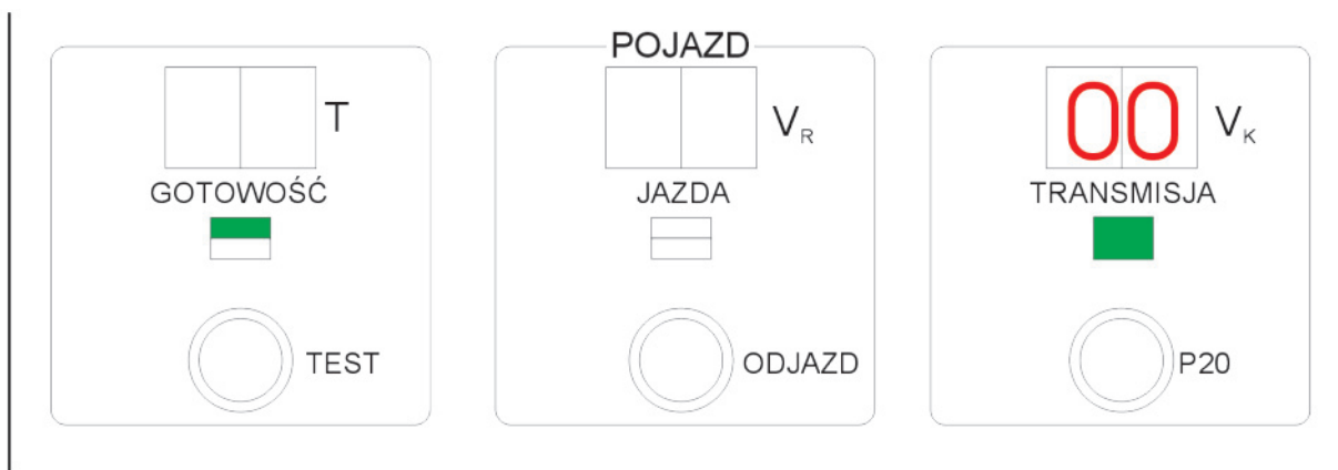
Rys. 39 Sygnał Sk O
