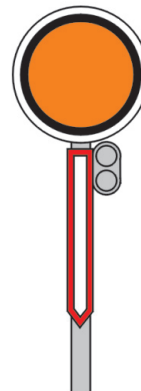
Rys. 33. Sygnał Ot 1 (dzienny)
