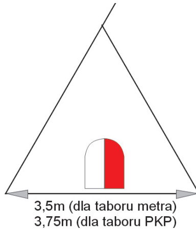
Rys. 56 Wskaźnik W 17
