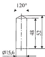
Rys. 2. Tłok cylindryczny z brązu, wymiary w mm
