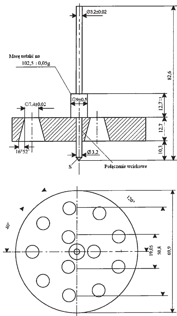
Rysunek 1 Penetrometr
