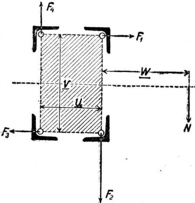
Rys. 1. (do § 36). Siły skręcające słup.
