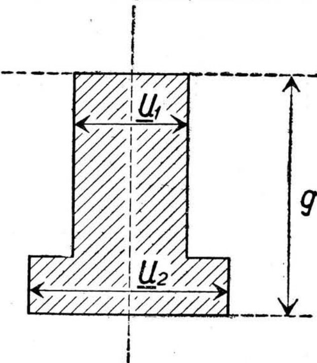
Rys. 2. Fundament betonowy słupa. (do § 52).
