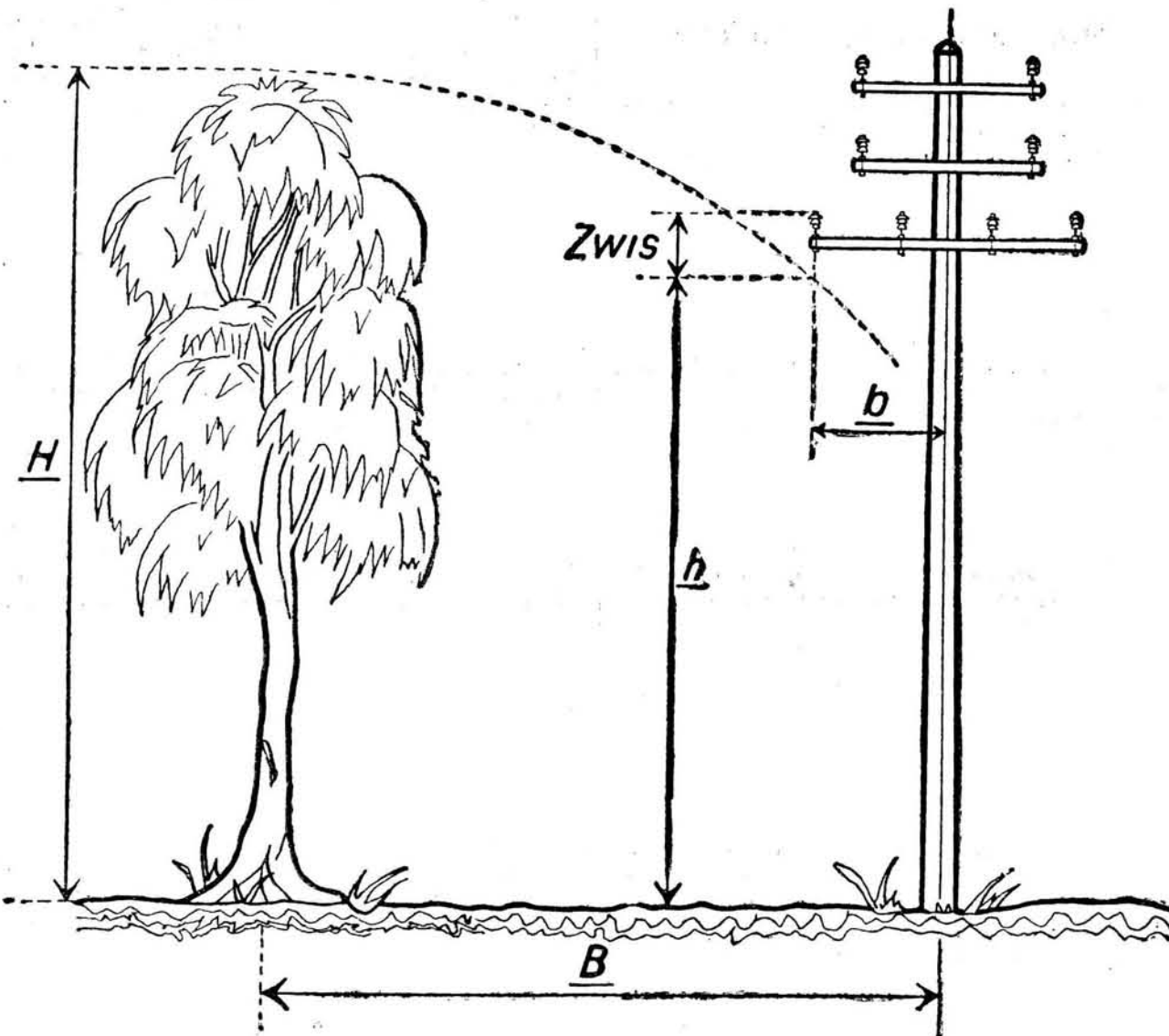
Rys. 1. (do § 69). Przejście przez las.
