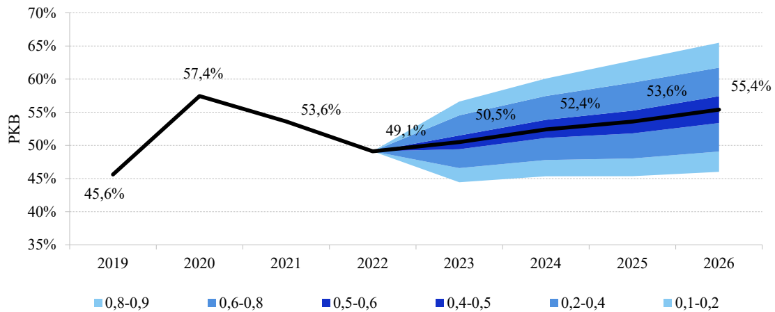
Wykres 8. Stochastyczne projekcje długu od 2023 roku
